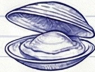
صفيحات الغلاصم
