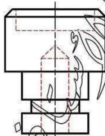
مسقط يساري
